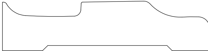
BASE CAP 23253 3/4" X 3 1/4" OLD 3125-1
